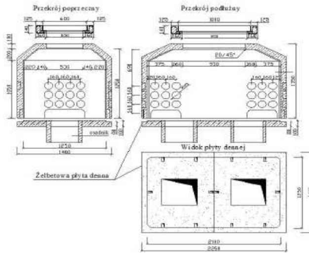
KONSTRUKCJA
